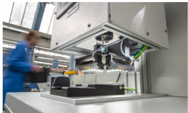
Verifikations-Station zur manuellen Qualitätskontrolle von Datamatrix Codes
