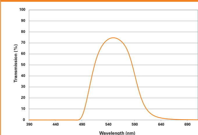
Objektivfilter BP 550nm (Art. Nr.: 303.0004.14)
